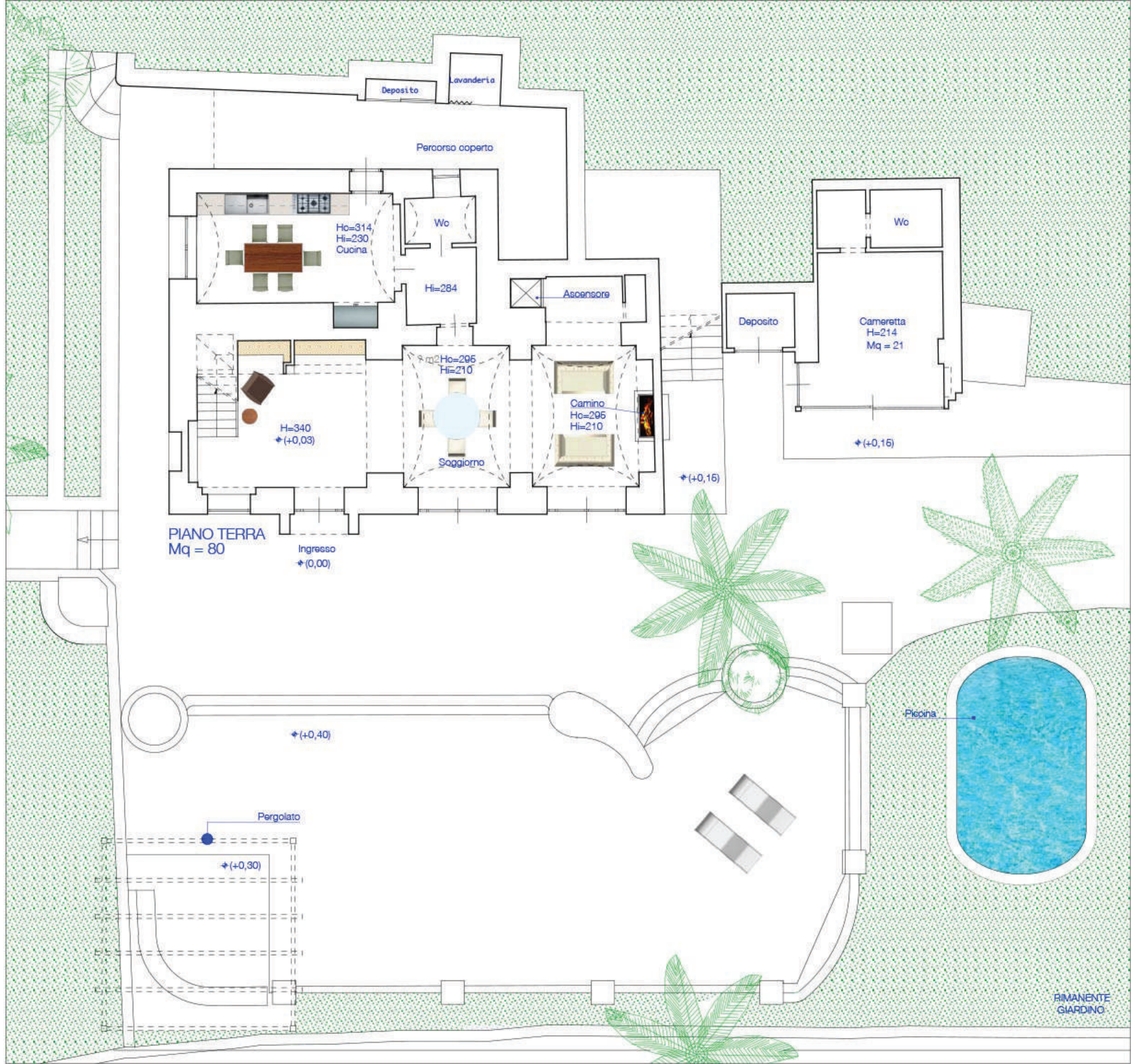
PIANTA PIANO TERRA STATO ATTUALE - SCALA 1:100
