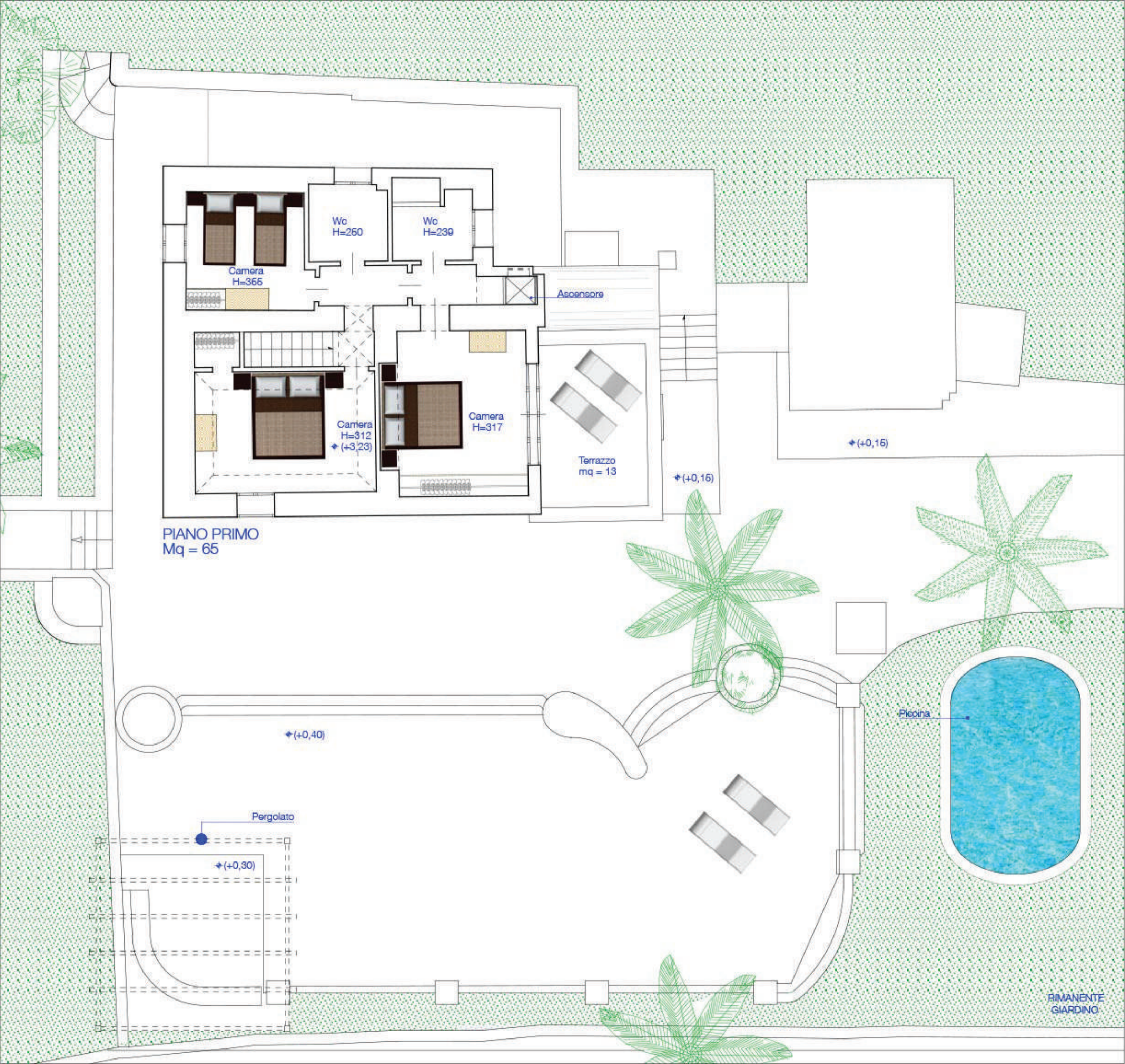
PIANTA PIANO PRIMO STATO ATTUALE - SCALA 1:100
