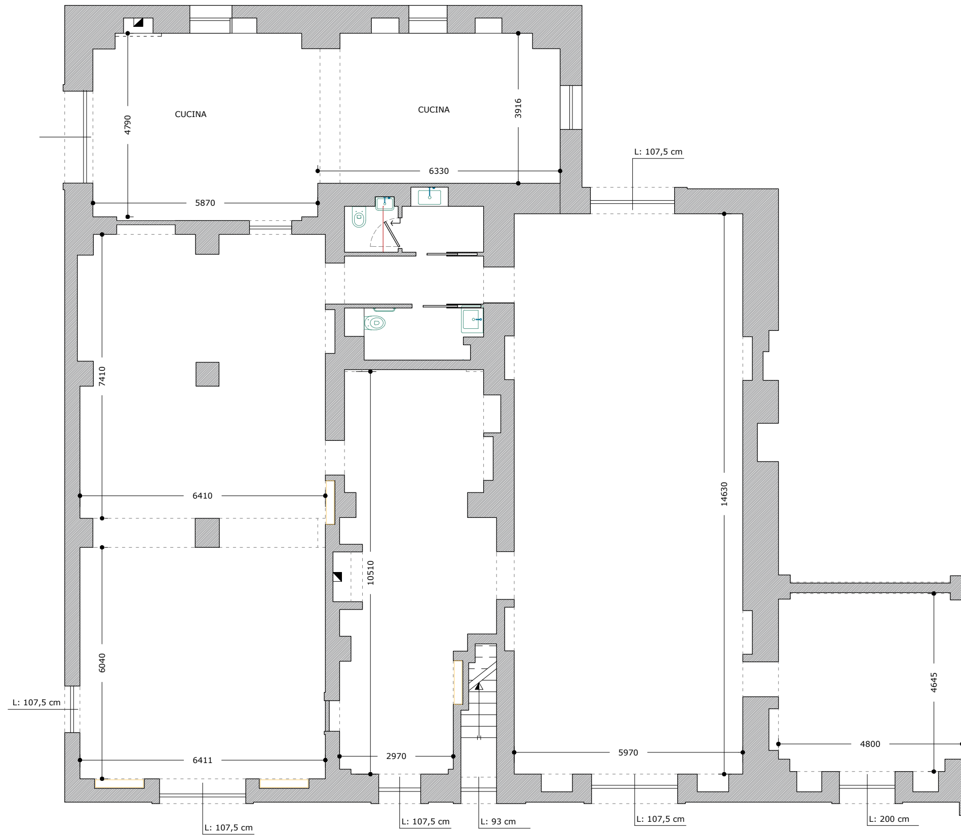
Planimetria Piano Terra - Scala 1:100
